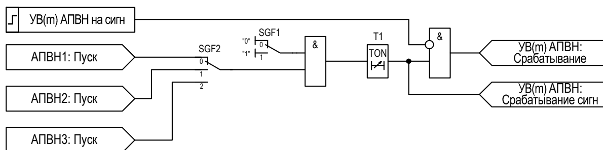
Рисунок 2.8 – Функциональная схема «УВ(м) АПВН»
